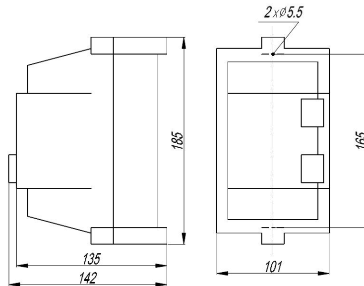
Рисунок Б.2-Пускатель ПМ12-025220 на номинальный ток 25А в пластмассовой оболочке.
