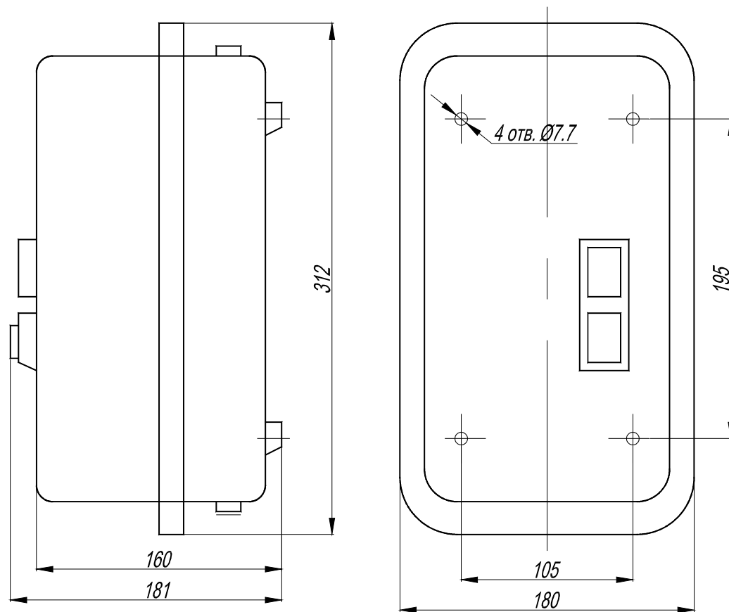
Рисунок Б.3- Пускатели ПМ12-040220, ПМ12-063220, ПМ12-100220 на номинальные токи 40, 63 и 100 А в металлической оболочке.
