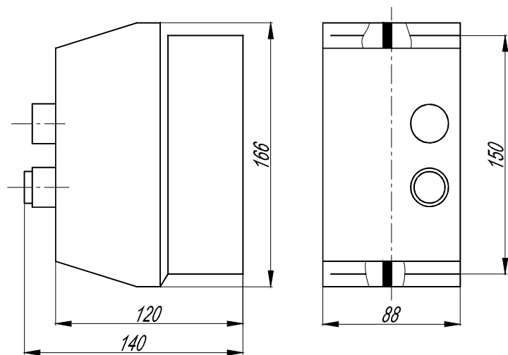
Рисунок Б.1- Пускатель ПМ12-010220 на номинальный ток 10А в пластмассовой оболочке.
